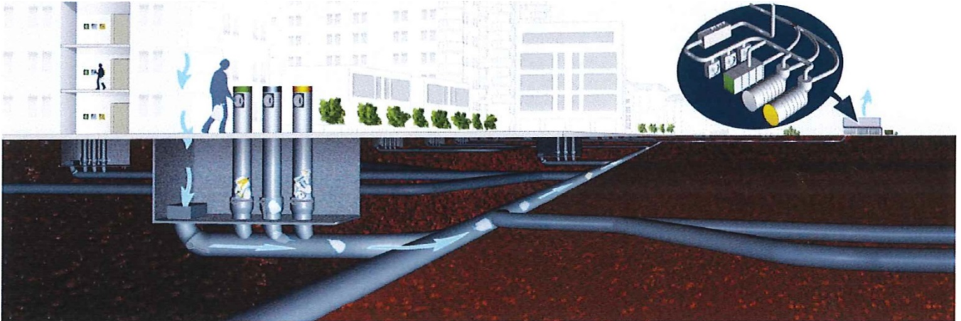
Schematisk beskrivning av sopsugssystemet
