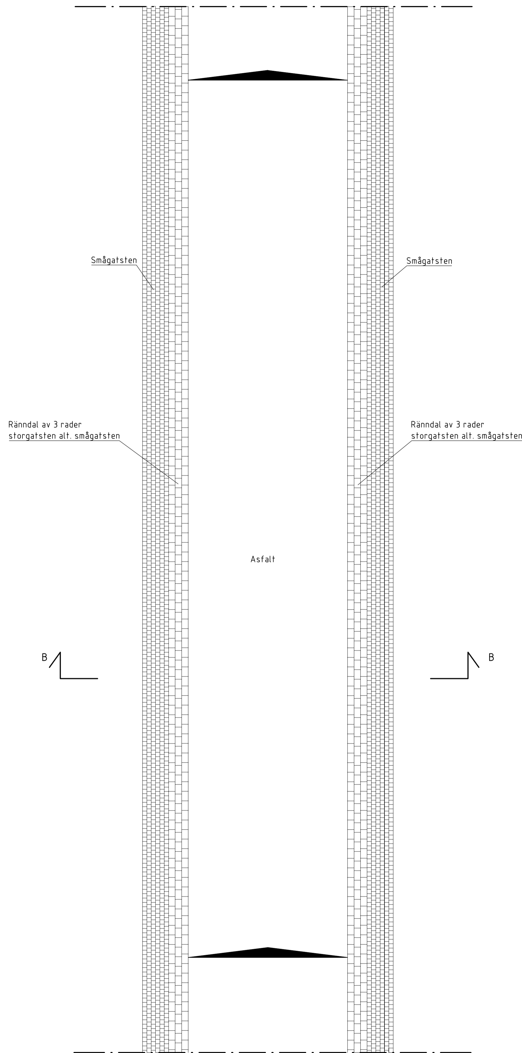
GRÄND 2 PLAN SKALA 1:50
