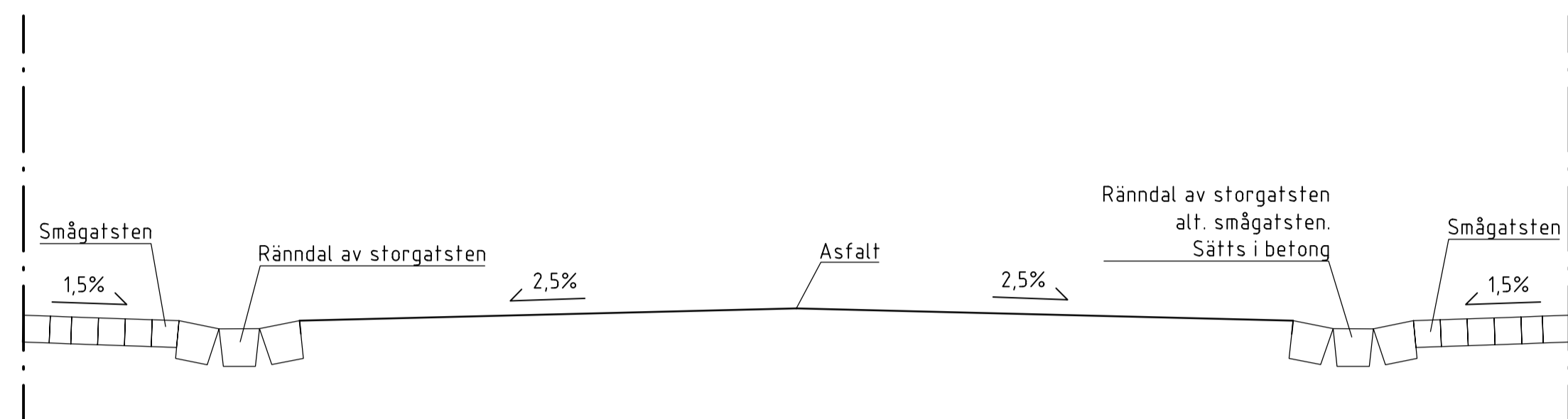
GRÄND 2 SEKTION B-B SKALA 1:20
