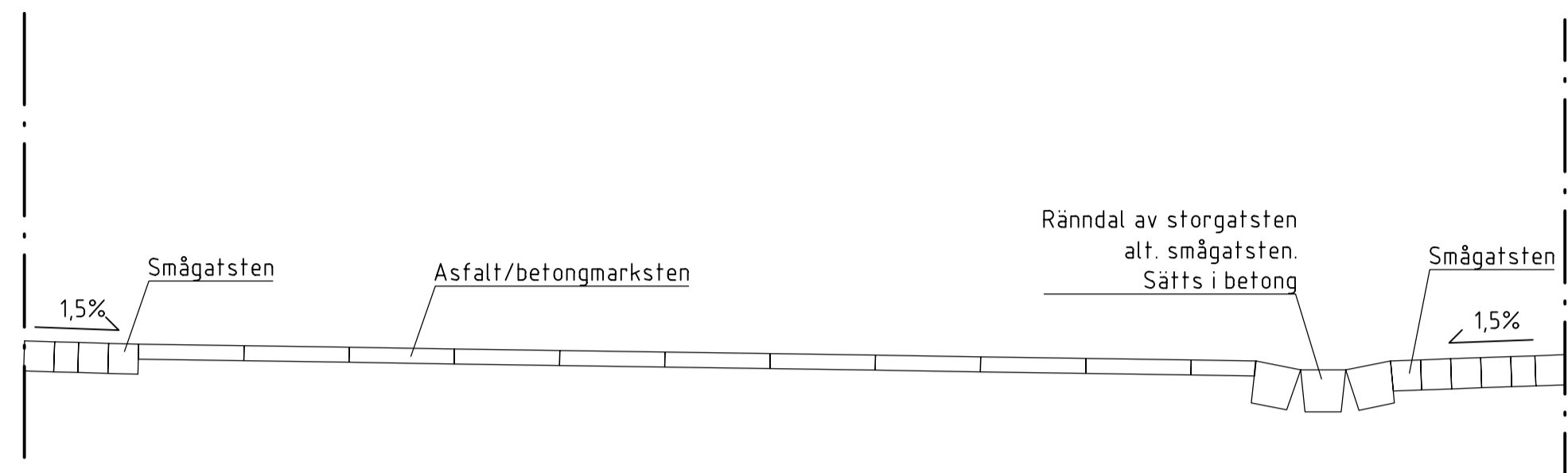
GRÄND 1 SEKTION A-A SKALA 1:20
