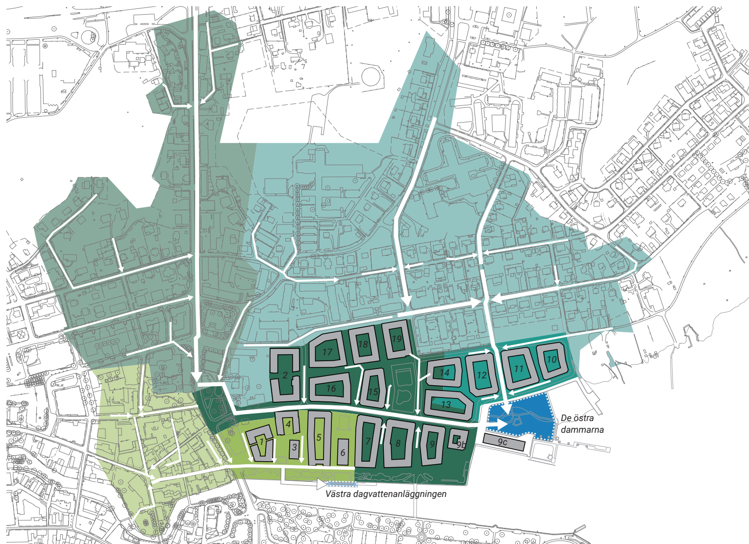
Figur 25. Diagram dagvatten
