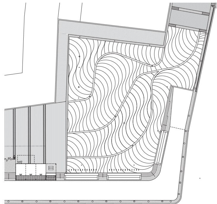
Figur 294. Beläggningssnitt för Hamnplan.
