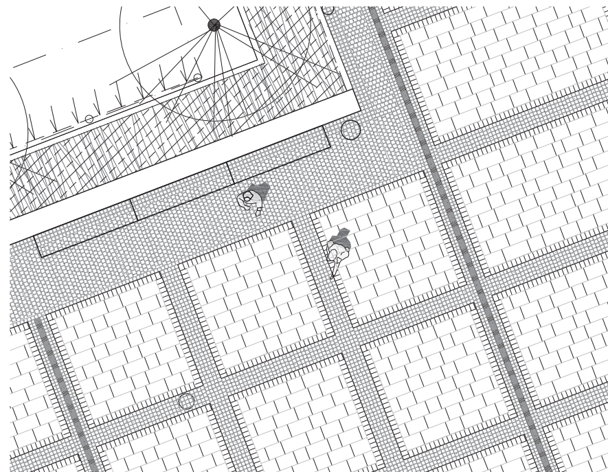
Figur 250. Beläggningssnitt Sjötullstorget och södra delen av Kärleksparken med ny parkering. Torgets yta binder samman Hamnpromenaden med befintlig stadskärna.
