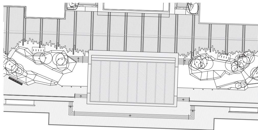
Figur 273. Beläggningssnitt "Bryggan" med södervända trappor som länkar samman det övre promenadstråket och de lägre bryggdelarna närmast vattnet. På "Bryggans" torg eftersträvas känslan av en parkett med sitt fiskbensmönster.
