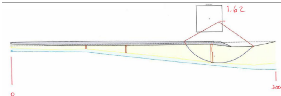
Figur 3 Beräkningssektion Brännäskilen (Pilgatan - Hamnbassängen)
