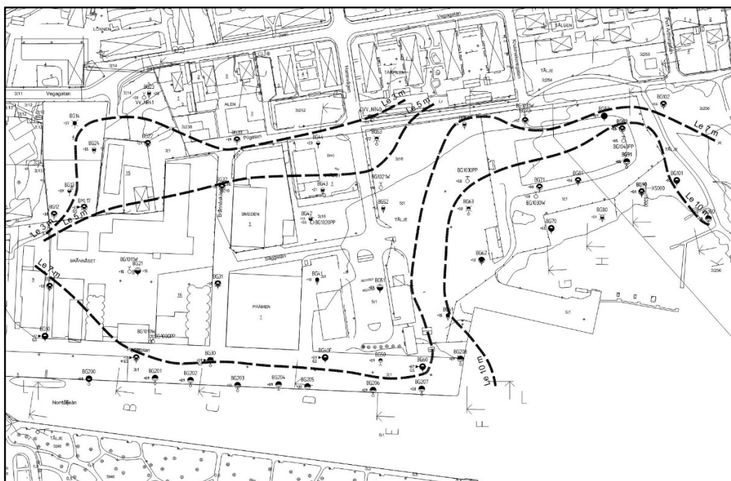
Figur 1 Schematiska lerdjupskurvor visande djup till underliggande lermorän
