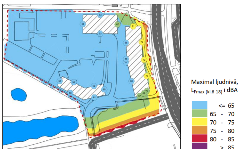
Figur 5. Beräknad maximal ljudnivå 1,5 m över mark för vägtrafik dag/kväll.
