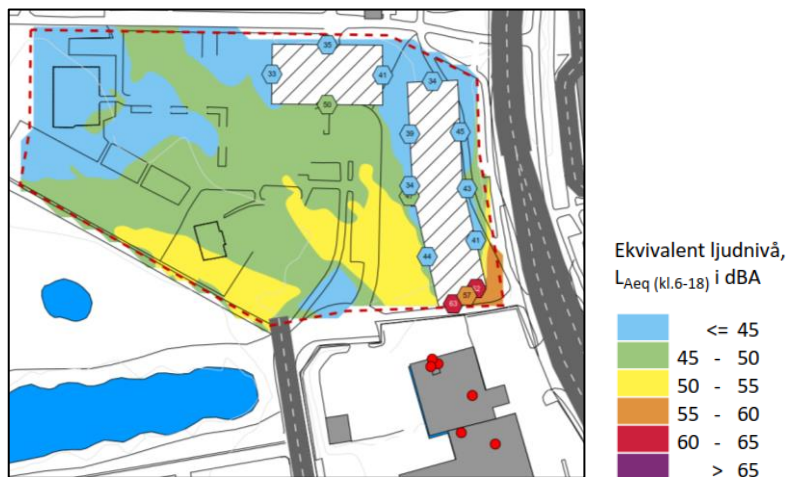
Figur 8. Beräknad ekvivalent ljudnivå 1,5 m över mark för verksamhetsbuller.
