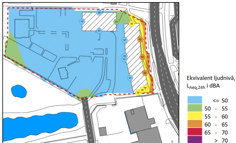
Figur 6. Beräknad ekvivalent ljudnivå 1,5 m över mark för vägtrafik.
