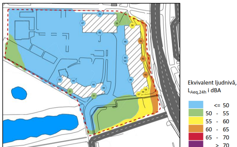
Figur 4. Beräknad ekvivalent ljudnivå 1,5 m över mark för vägtrafik.
