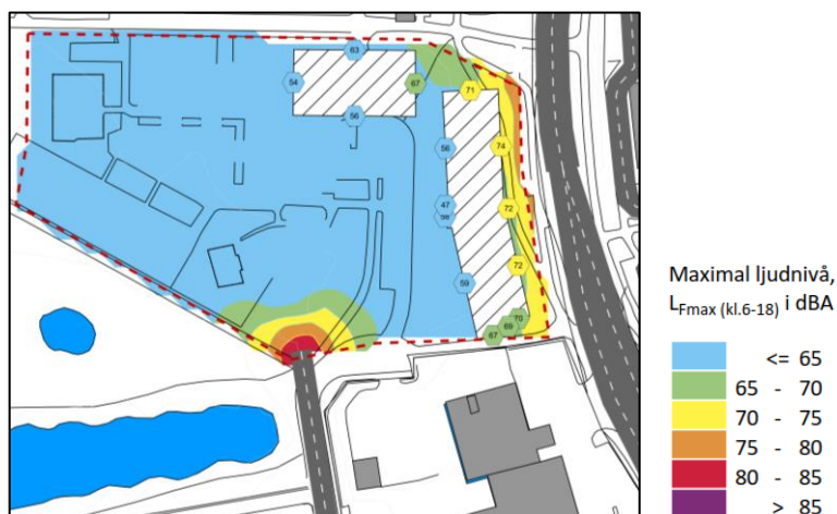
Figur 7. Beräknad maximal ljudnivå 1,5 m över mark för vägtrafik dag/kväll.
