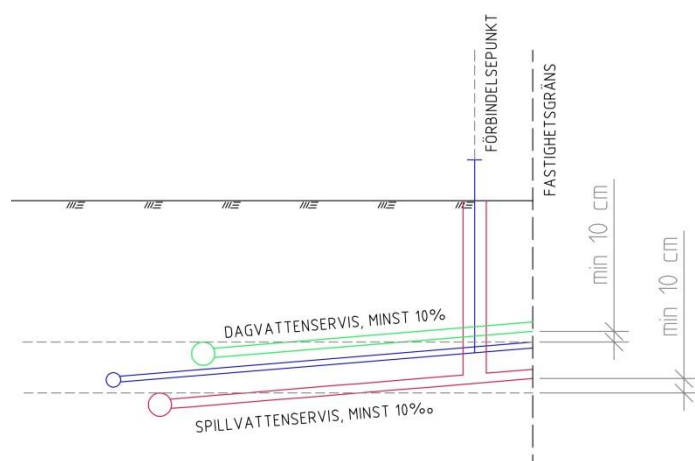
Figur 4. Vattengång på servisledning i fastighetsgräns
