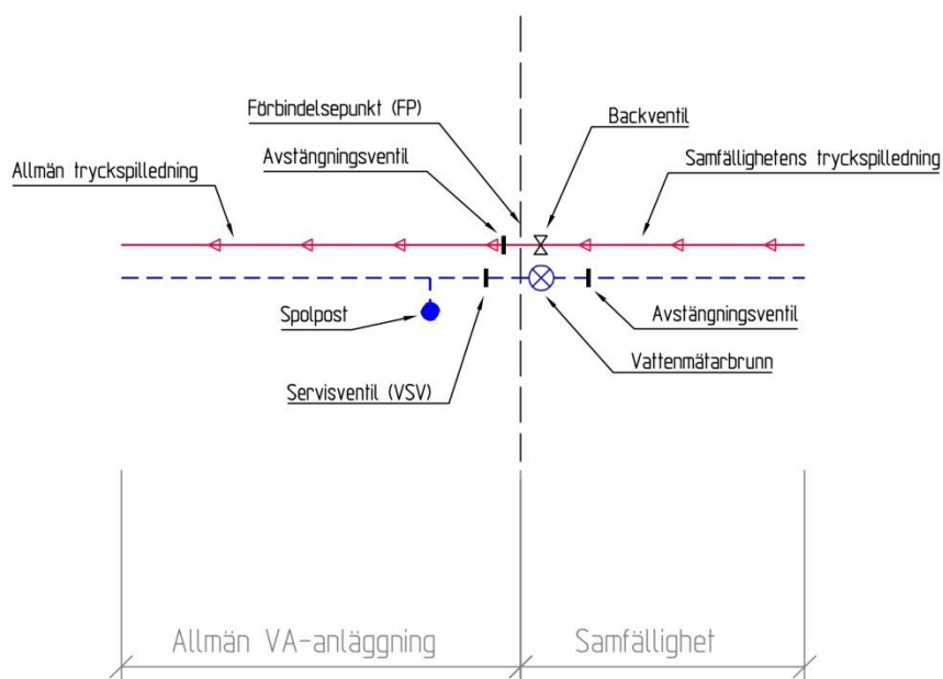
Figur 7. Anslutning samfällighet mot allmän tryckspilvattenledning.
