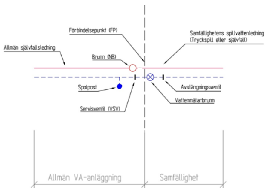
Figur 6. Anslutning samfällighet mot allmän självfallsledning.
