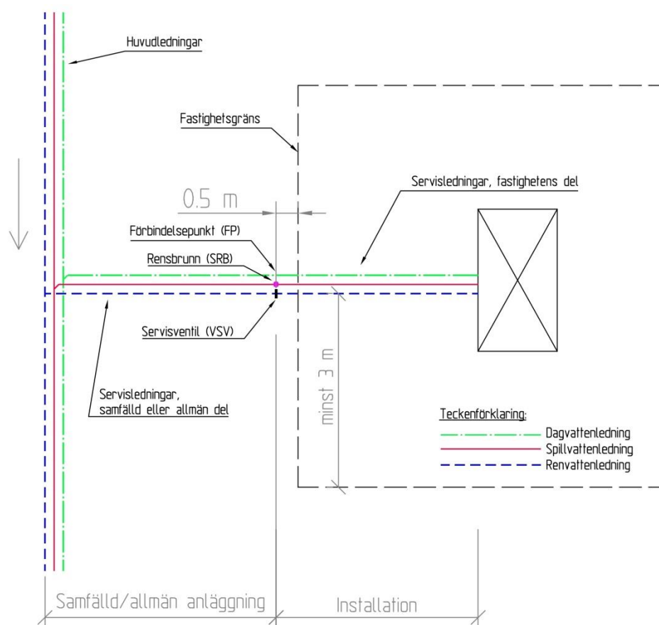
Figur 2. Servisanslutning självfall
