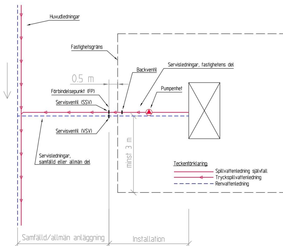
Figur 3. Servisanslutning LTA-system
