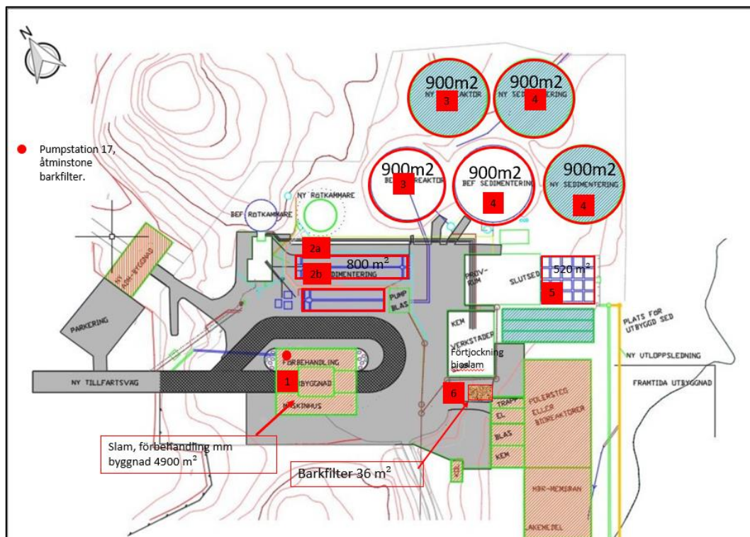
Figur 5-1. Skiss över det planerade reningsverket och identifiering av utsläppspunkter.
