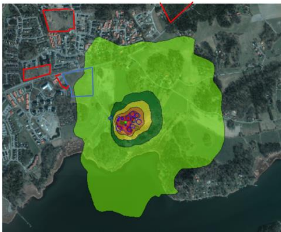
Figur 6-3. Resultat av modelleringen med planerade och beslutade detaljplaner markerade i rött och pågående planskiss markerat i blått. Det pågående planskissområdet nordväst om reningsverket hamnar innanför området med 2-3 luktenheter.
